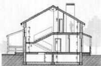
Разрез 1-1
